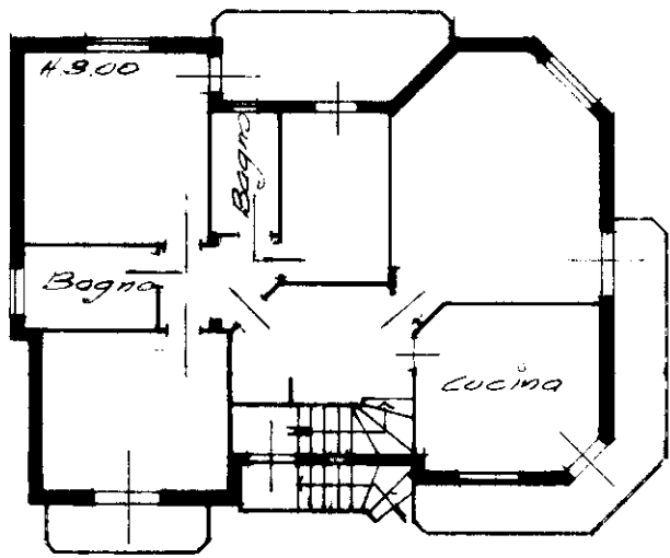
PIANO PRIMO
